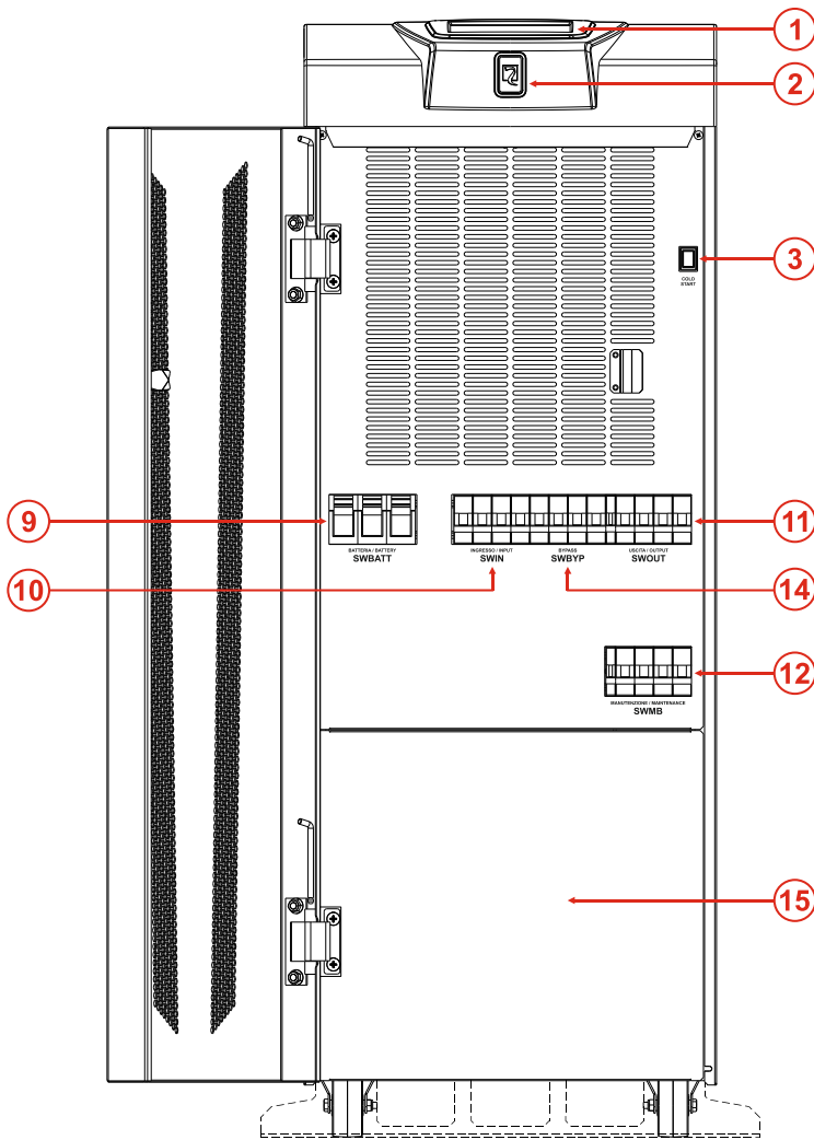
ВИД СПЕРЕДИ
