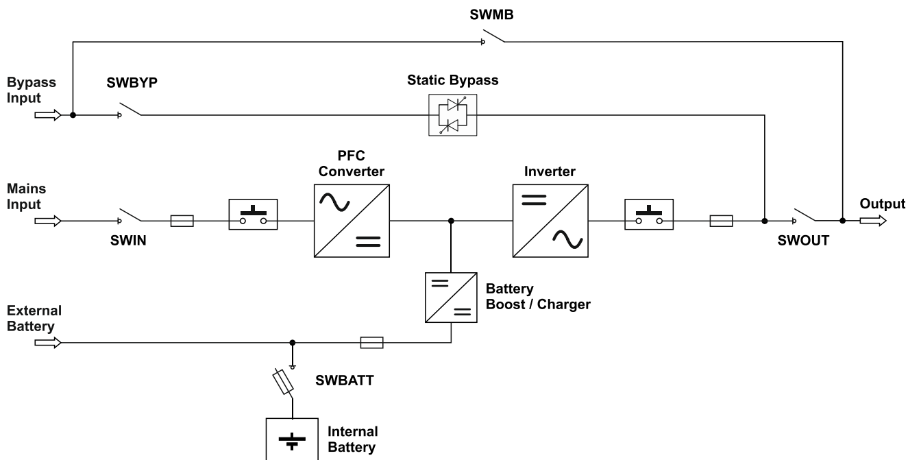
Блок-схема ИБП с двойным вводом (с отдельным байпасом)
