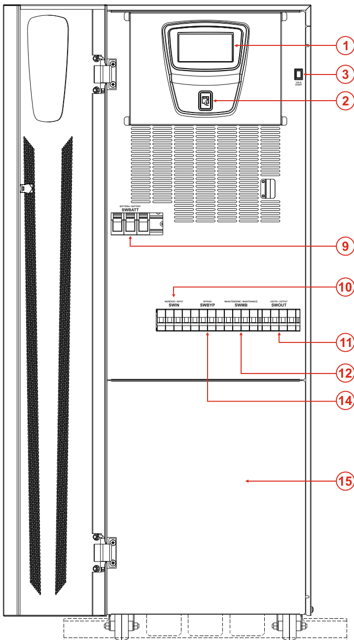
ВИД СПЕРЕДИ
