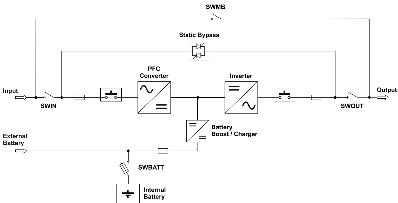
Блок-схема ИБП с одним вводом (без отдельного байпаса)
