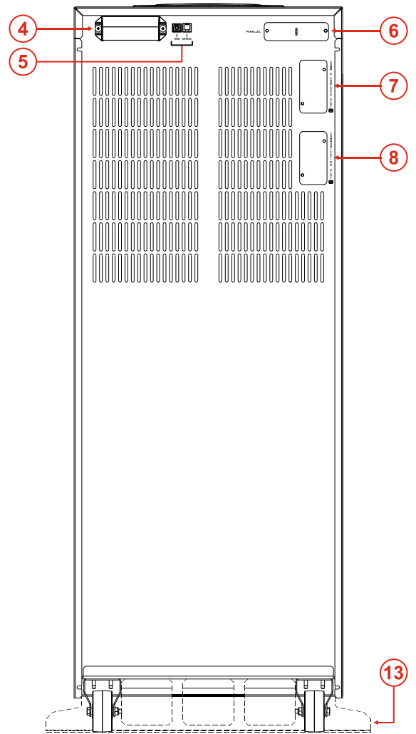
ВИД СЗАДИ
